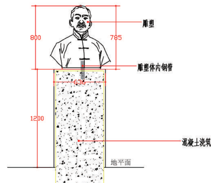
雕塑基础及预埋件示意图一立面
