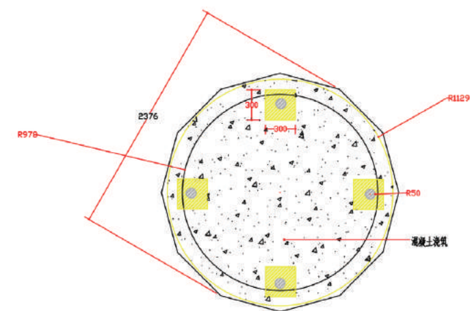
雕塑基础及预埋件示意图—平面
