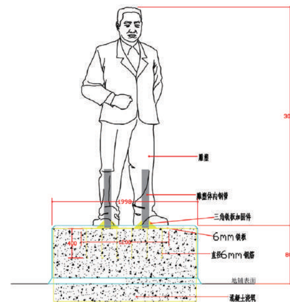
雕塑基础及预埋件示意图—立面
