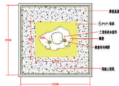
雕塑基础及预埋件示意图—平面
