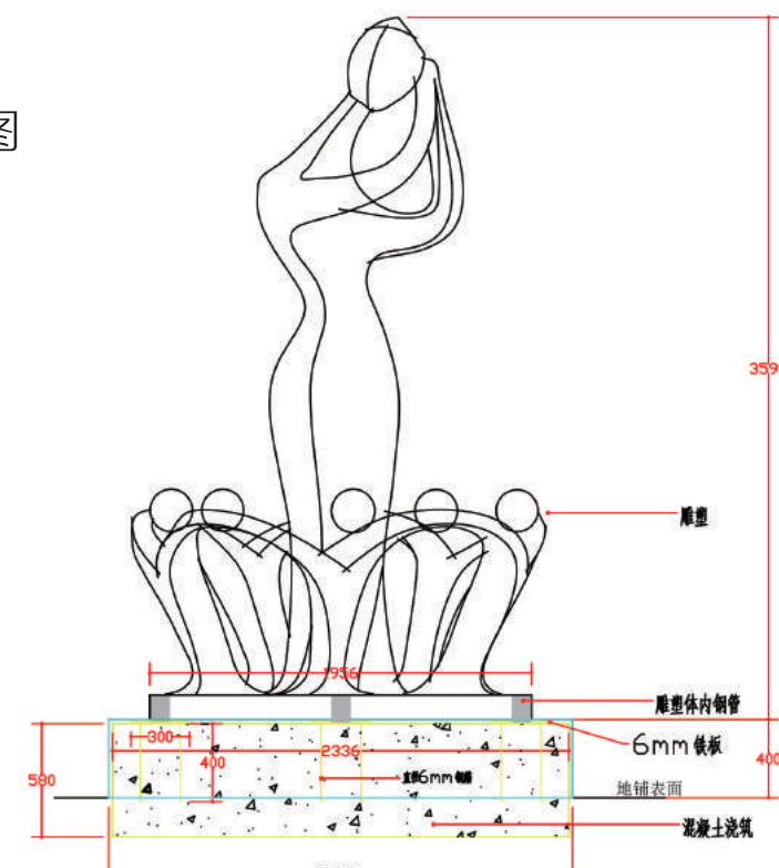
雕塑基础及预埋件示意图—立面
